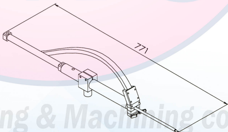
Air rod feeder
